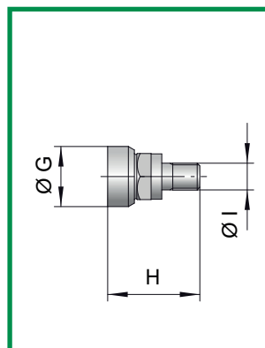
可互换插件
